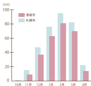
最深積雪平均値 (平成2年～令和2年 気象庁)
